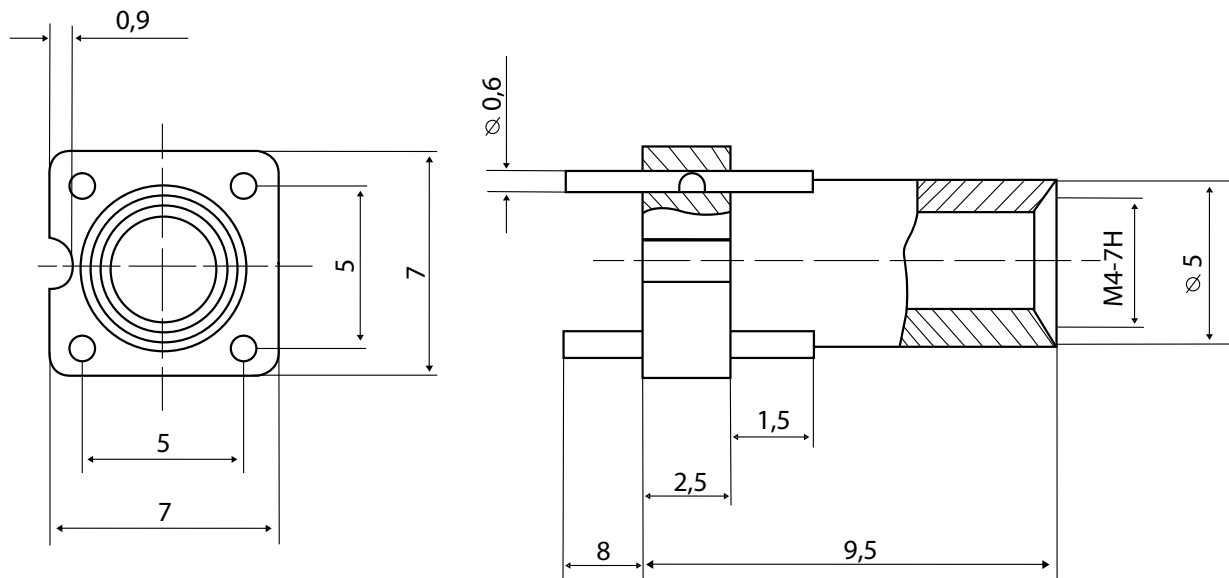
Габаритный чертеж
