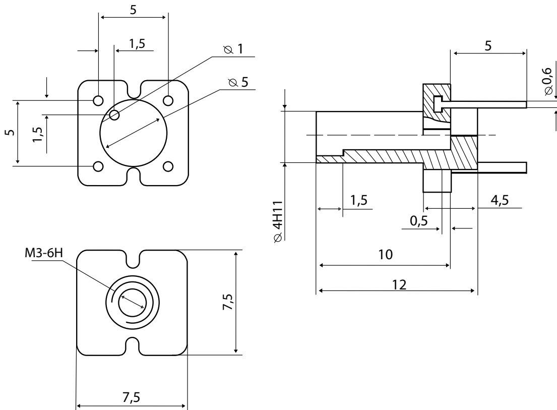
Габаритный чертеж
