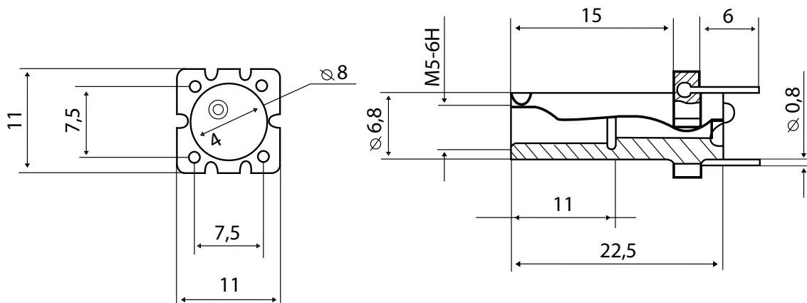
Габаритный чертеж
