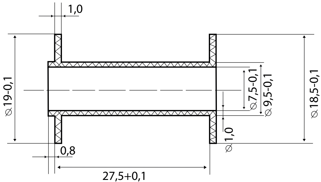
Габаритный чертеж
