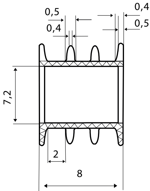
Габаритный чертеж
